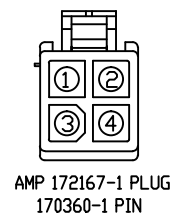
MOTOR CONNECTOR 접속도
